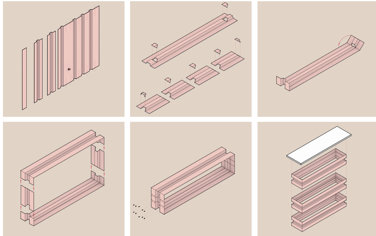
Verarbeitungsprinzip der Blechtre
